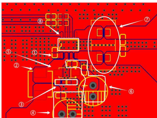
顶层
